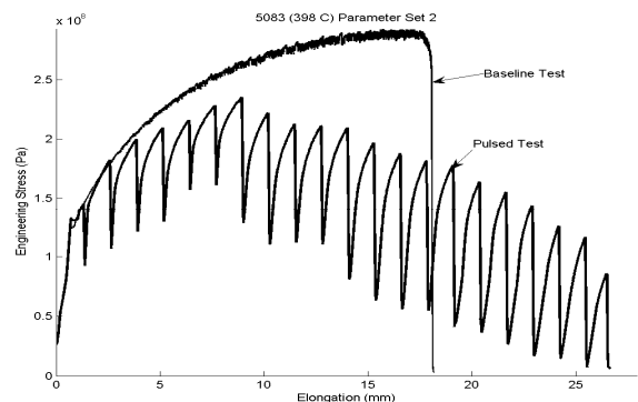
FIGURE 20 - 5083 - 398°C - PARAMETER SET 2
